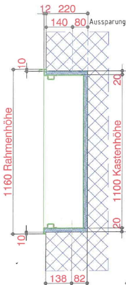
Vertikalschnitt
