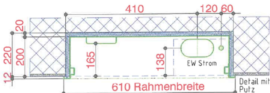
Grundriss Unterseite
