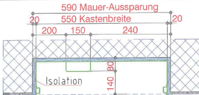
Grundriss Oberseite
