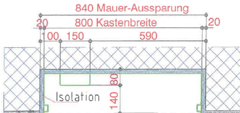
Grundriss Oberseite
