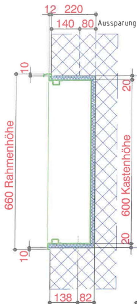
Vertikalschnitt
