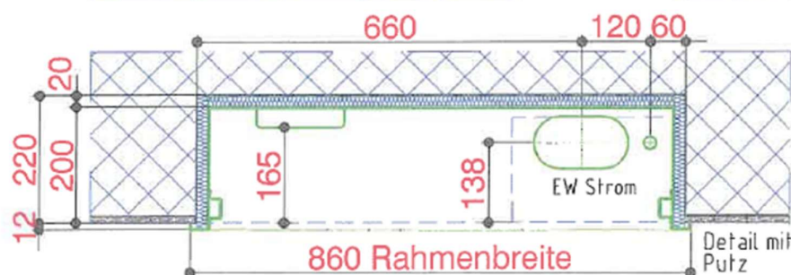
Grundriss Unterseite
