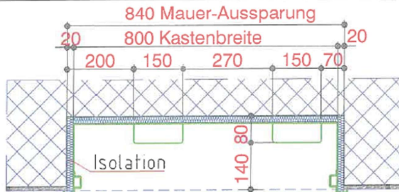
Grundriss Oberseite
