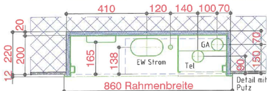
Grundriss Unterseite
