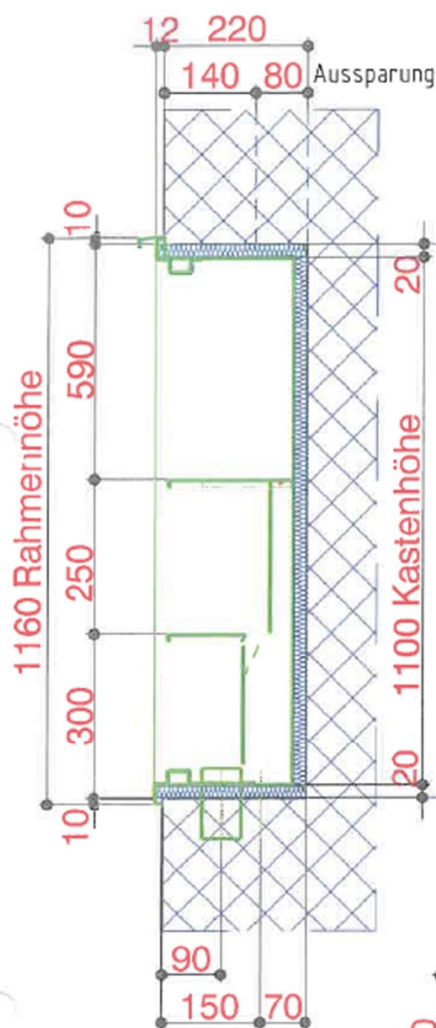
Vertikalschnitt
