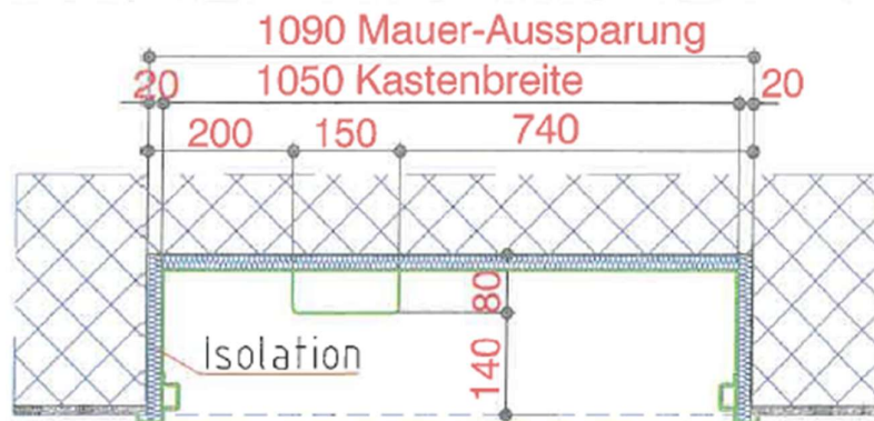
Grundriss Oberseite
