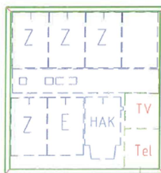
Grundriss Unterseite
