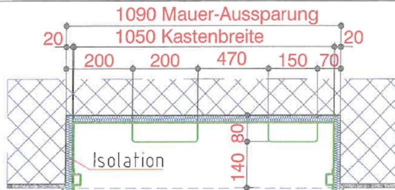
Grundriss Oberseite
