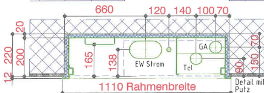
Grundriss Unterseite
